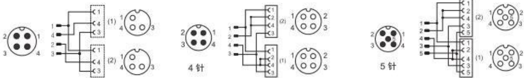
T2 电路示意图
