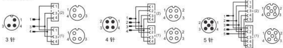
T1 电路示意图
